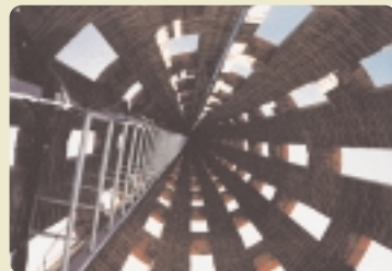
ELADIO DIESTE, TORRE PER TRASMISSIONI TELEVISIVE A MALDONADO (URUGUAY) SCALA DI SERVIZIO
